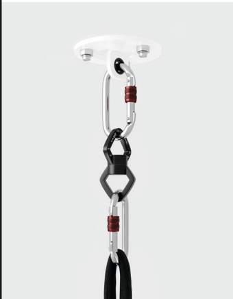
PLATTE MIT DÜBELN IN DER DECKE
