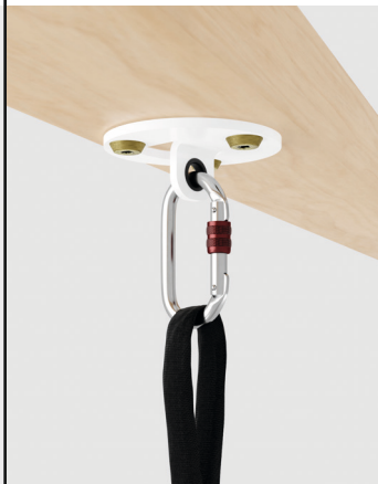
PIASTRA CON VITI NELLA TRAVE
